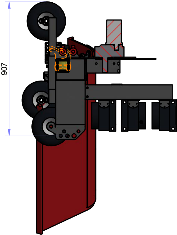
A-A ( 1 : 15 )
