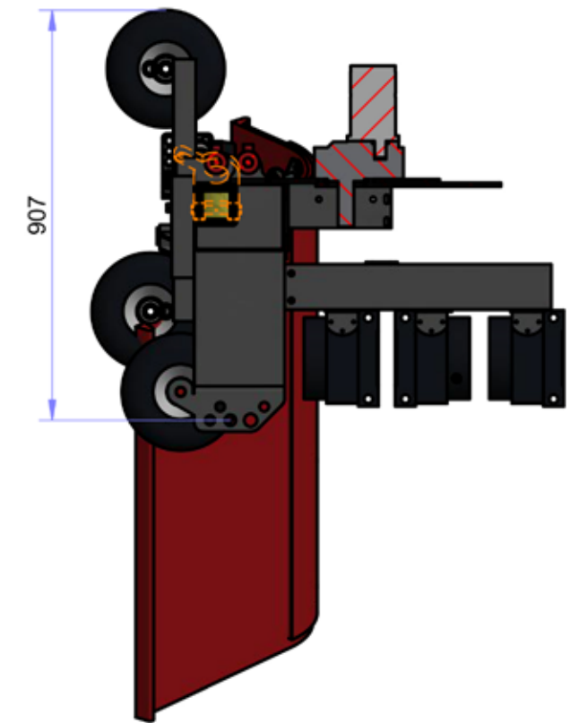
A-A ( 1 : 15 )
